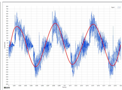
Abbildung 5: Differenzstrom mit einer Grundschwingung von 250 Hz
